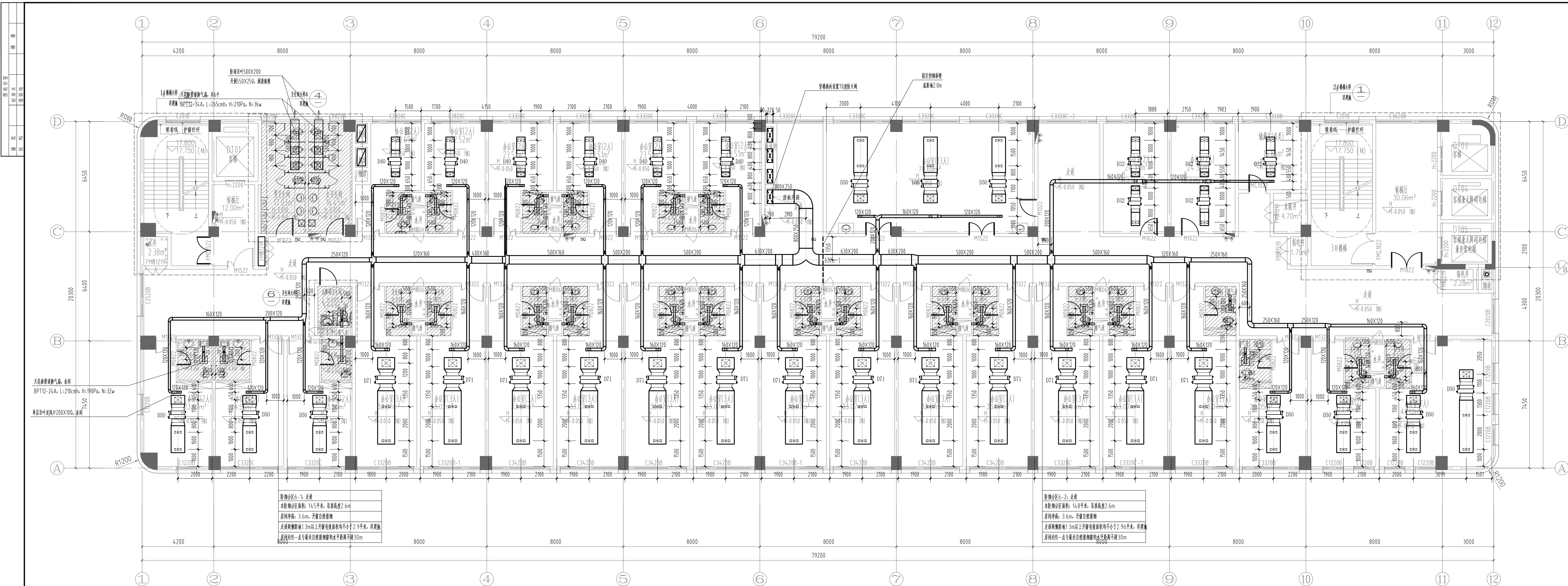
六层通风、防排烟、空调平面图 1:100
