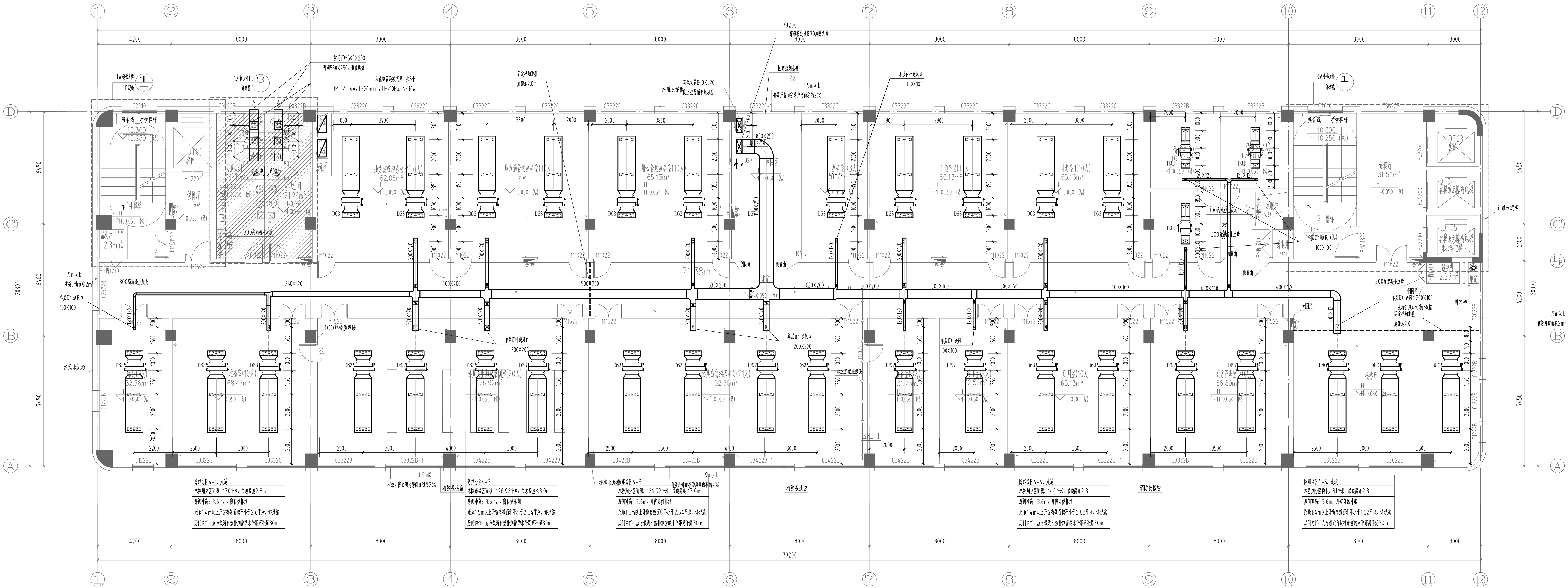
四层通风、防排烟、空调平面图 1:100
