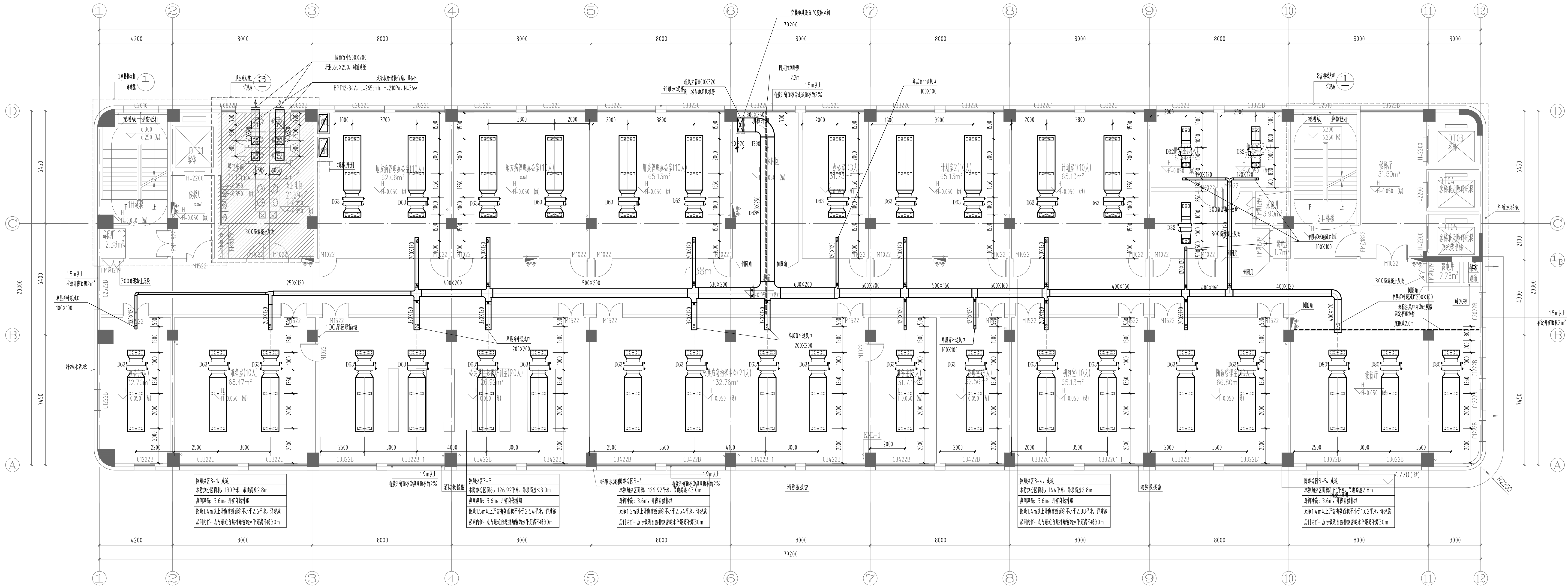
三层通风、防排烟、空调平面图 1:100
